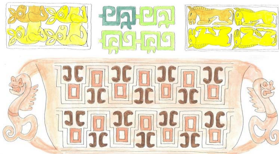
7. ábra. Matematika a kelet-ázsiai művészetekben.
