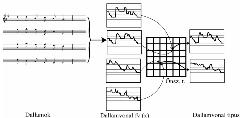
2. ábra. Az önszervező térkép. A hasonló dallamokból származtatott dallamvonal függvények (számsorok) a rács egy adott pontján átlagolódnak a tanulási folyamatban. Így keletkeznek a dallamvonal típusok.
