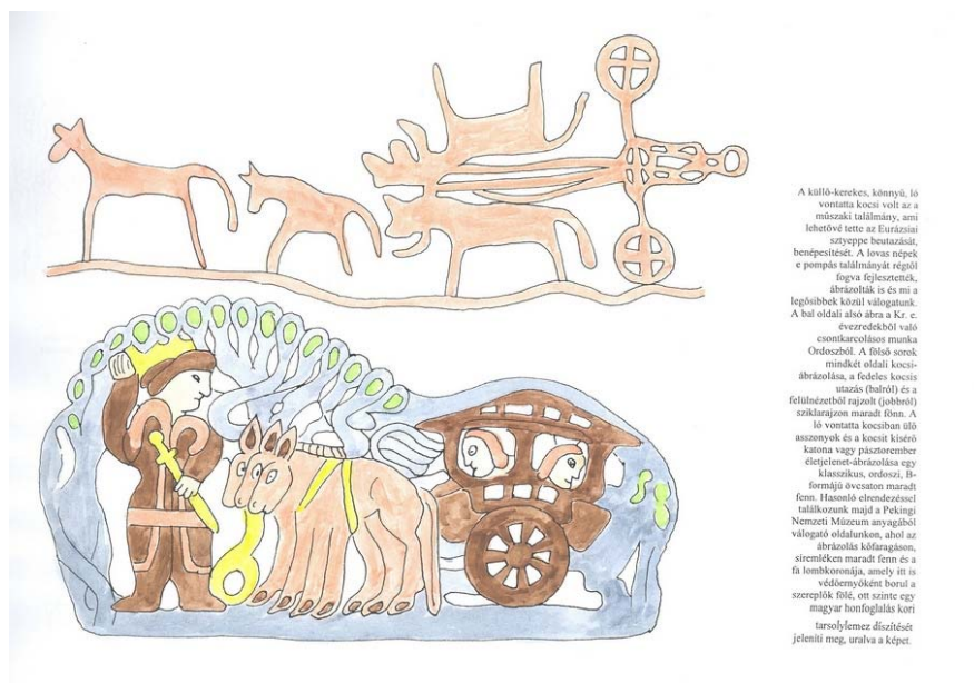
8. ábra. Eurázsiai lovasnépek kocsizása 3000 évvel és 2000 évvel ezelőtt.
