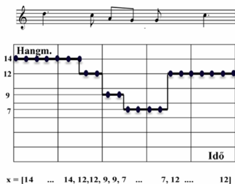
1. ábra. A dallamvonalat leíró vektor származtatása. A hangmagasság-idő függvényből a pontokban veszünk mintát, és ezeket az \underline{x} vektorban tároljuk. A vektor dimenziószáma a minták számával egyenlő.
