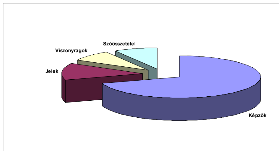
1. ábra A szavakkal végzett nyelvi műveletek aránya a magyar nyelvben
