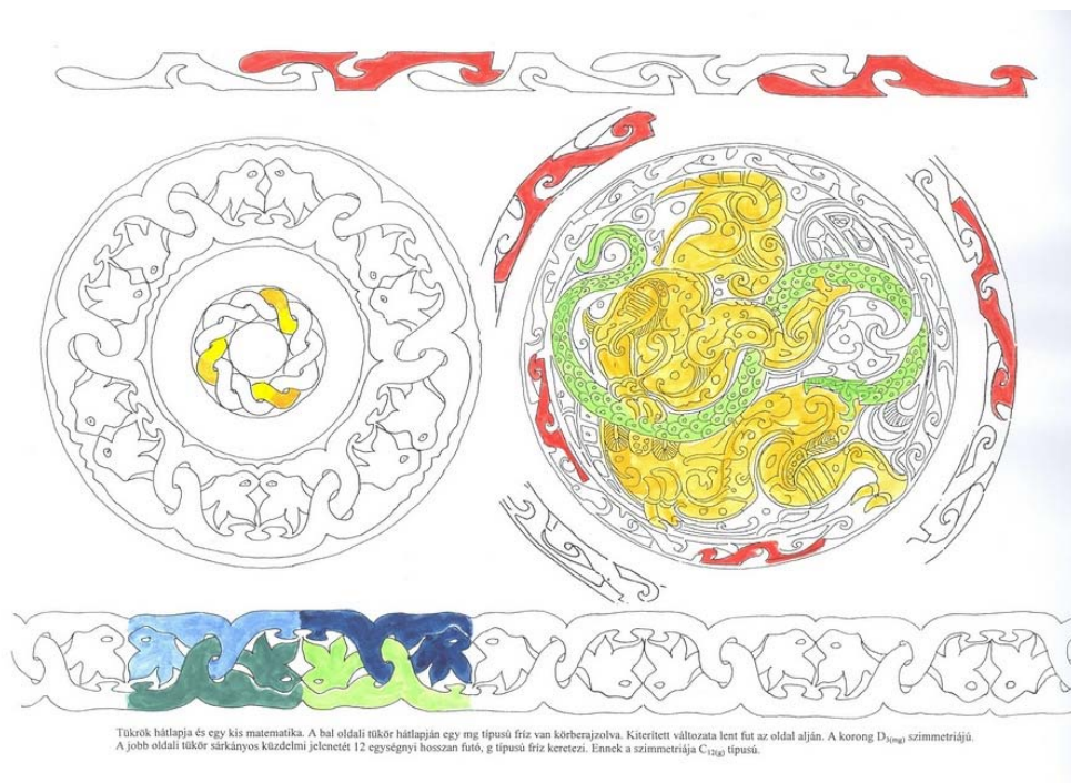
4. ábra. Érdekes matematikájú tükrőhátlapi díszítések: balra D_{3(mg)} , jobbra C_{12(g)} peremmel.
