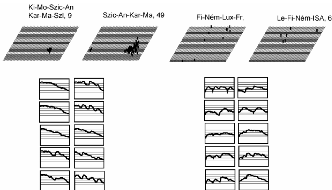
5. ábra. Bal: A keleti mag típusai az ősnyelv térképén, néhány jellemző dallamvonallal.
