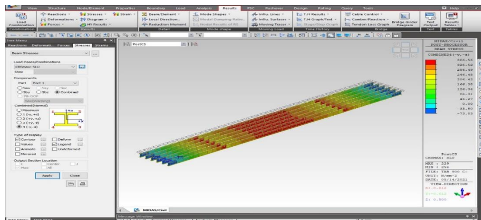
3.7. ábra Max feszültség az alsó övben ULS állapotban S=366,56 N/mm² ( <460/1,1=418,20 N/mm²)
