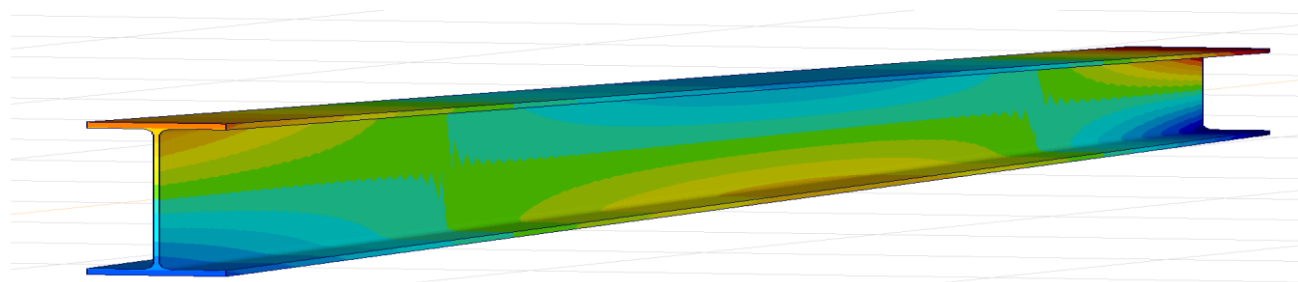
2.2. ábra Rúdszerkezeteknél normál feszültségek keresztmetszeten belüli eloszlásának megjelenítése látványterven.
