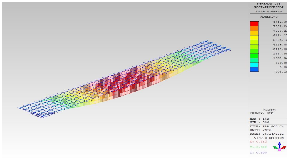
3.6. ábra Max forgatónyomaték ULS állapotban, a szélső tartón M_{max}=8781,30 kNm
