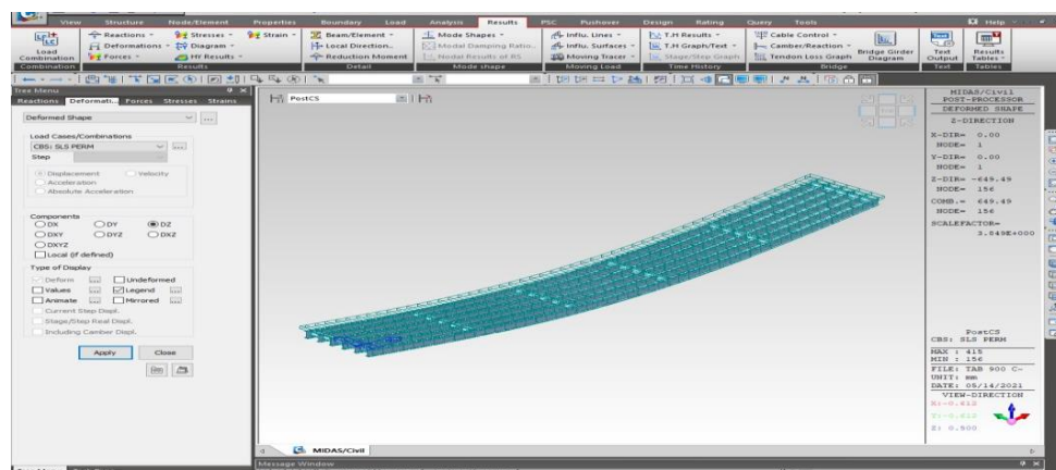
3.8 ábra A felszerkezet lehajlása önsúlyból és feszítésből SLS terhelésnél f_{1max}=649,49 mm
