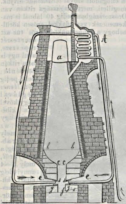
Olvasztó kemence.
