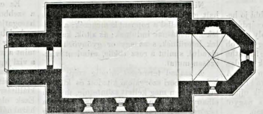
A veleméri templom alaprajza.
