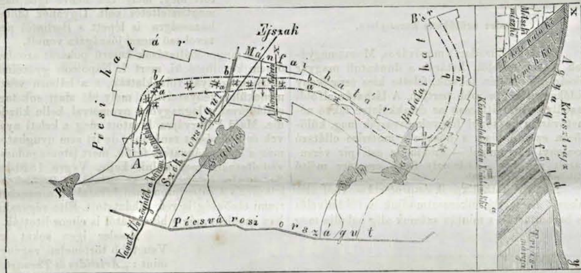
a) Alaprajz. b) Keresztmetsz.
