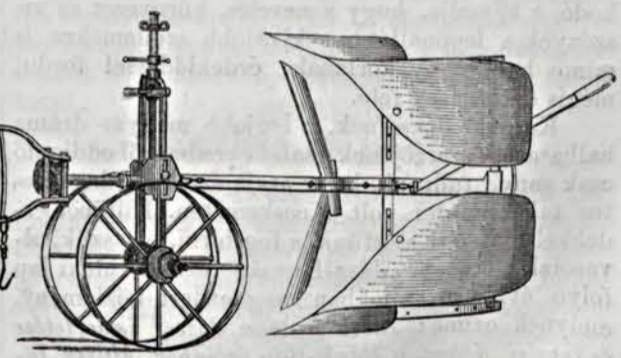
(9. ábra) Francia forgató-ekék.
