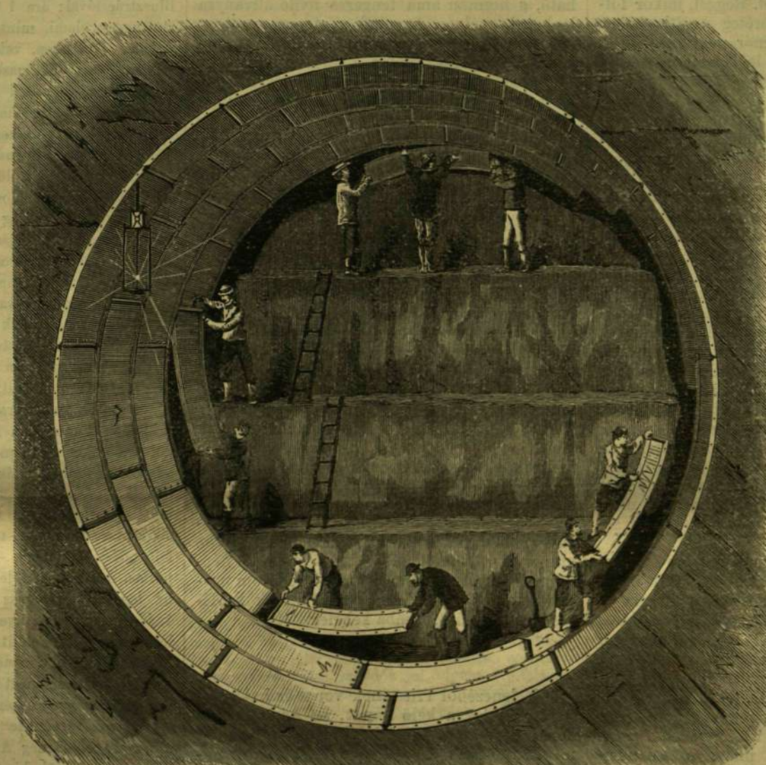
A KIVÁLT AKNA BEBORÍTÁSA PLÉHHEL. ALAGUT-ÉPÍTÉS A HUDSON FOLYÓ ALATT.
