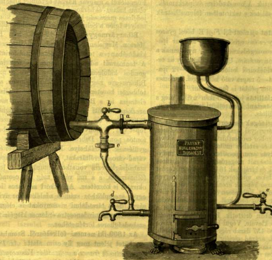
Készülék a bornak saját hordójában hevítésére.
