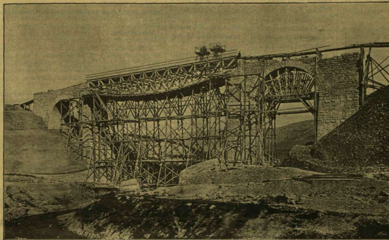
A HUKLIVAI VÖLGY ÁTHIDALÁSA.
