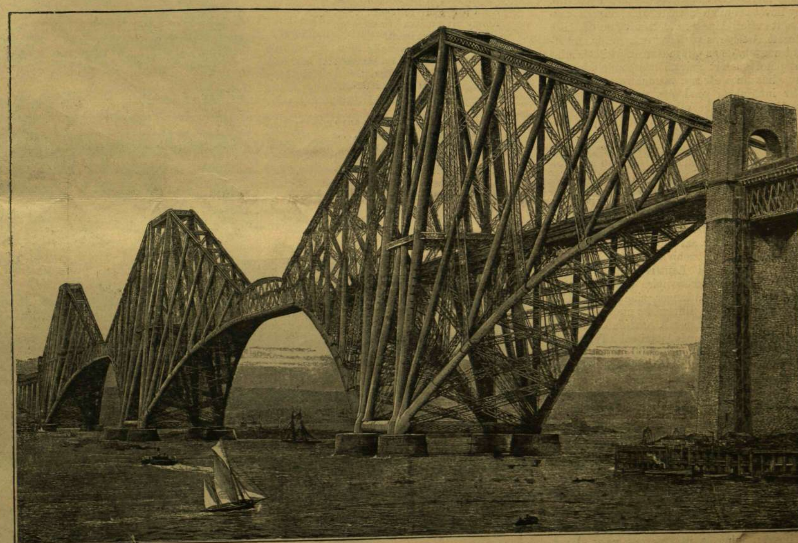
A FORTH-HID SKÓCZIÁBAN. — (MEGNYITATTOTT 1890. MÁRCIUS 4-ÉN.)
