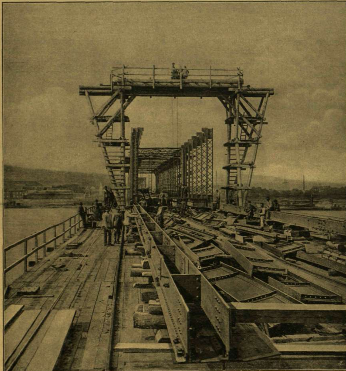
A POZSONYI ÚJ DUNA-HID. — Az épülő híd 5-ik modernnyílása, szerelés közben.
