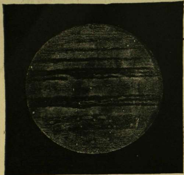
Jupiter még élete kezdetén van; nem látunk belőle úgyszólván mást, mint gőzöket és felhőket.
