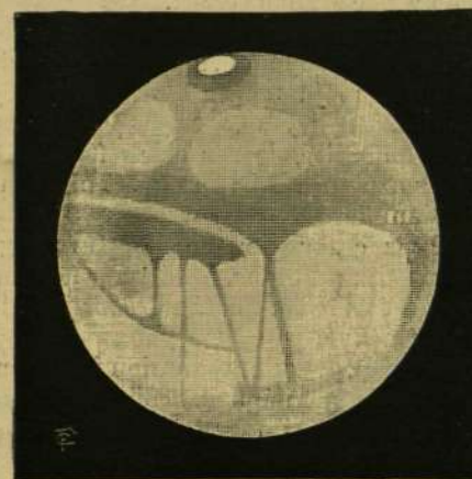
A Mars bolygó csak csekély kiterjedésű földközi tengerek képét mutatja.
