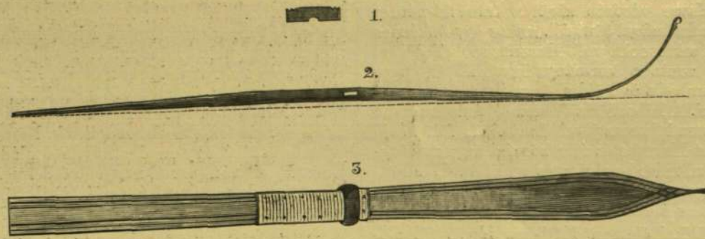
1. ábra. Kristianiai lábszánkó: 1. Átmetszet. 2. Oldalról nézve. 3. Felülről nézve.
