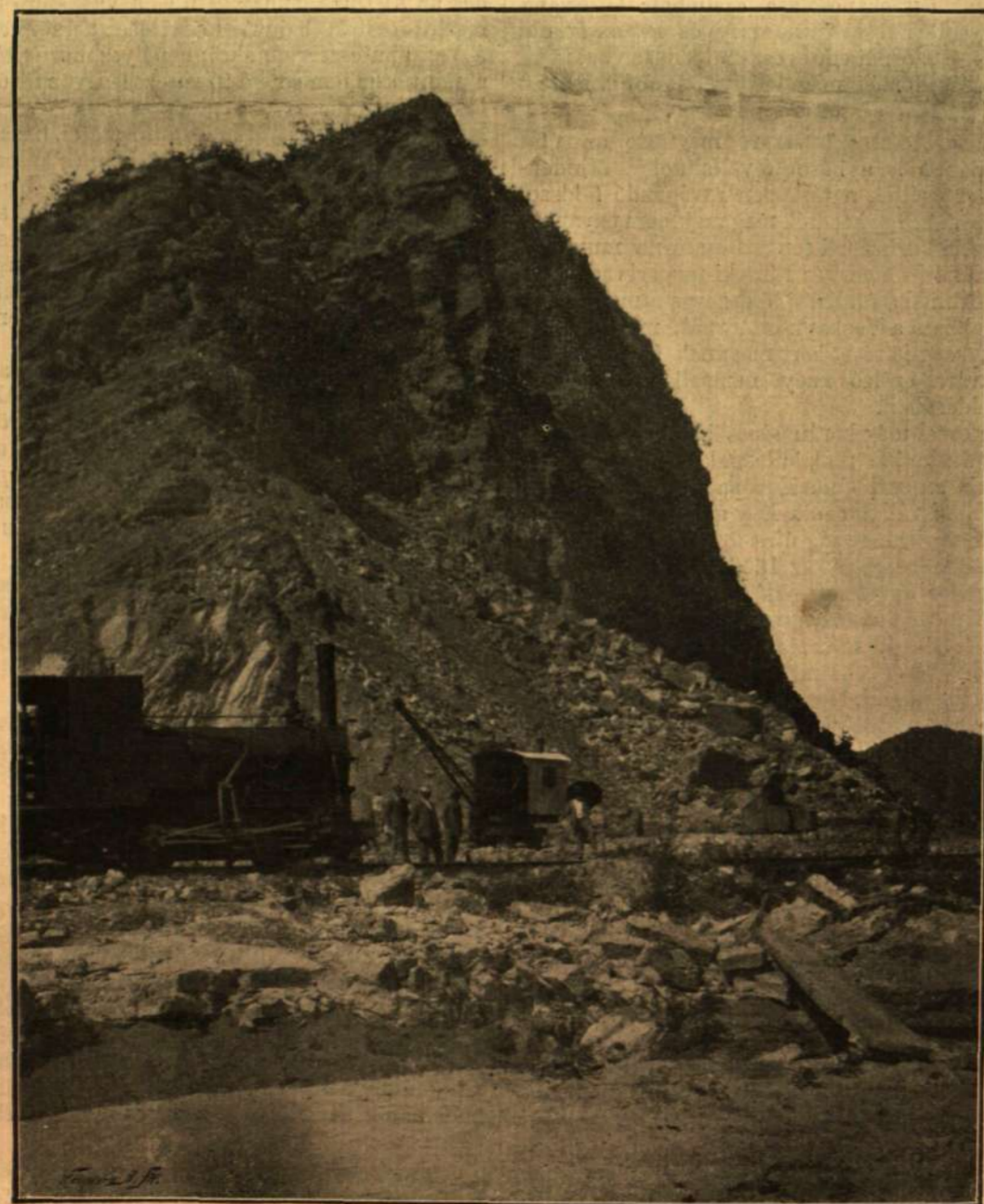
AZ AL-DUNÁRÓL. — A Greben-hegy a robbantási munkálatok közben.
