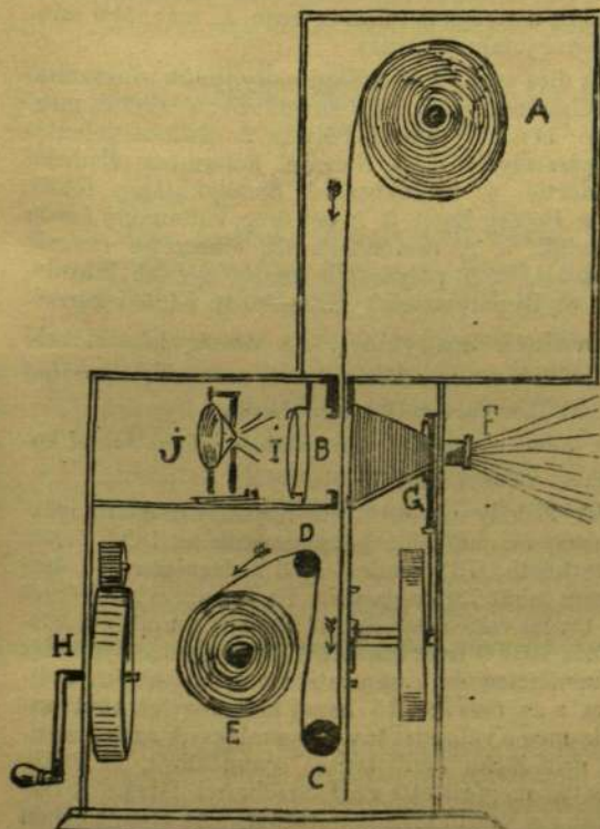
A KINEMATOGRAF ÁTMETSZETE.
