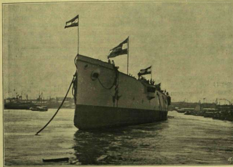
A Zenta a vizrebocsátás után.
