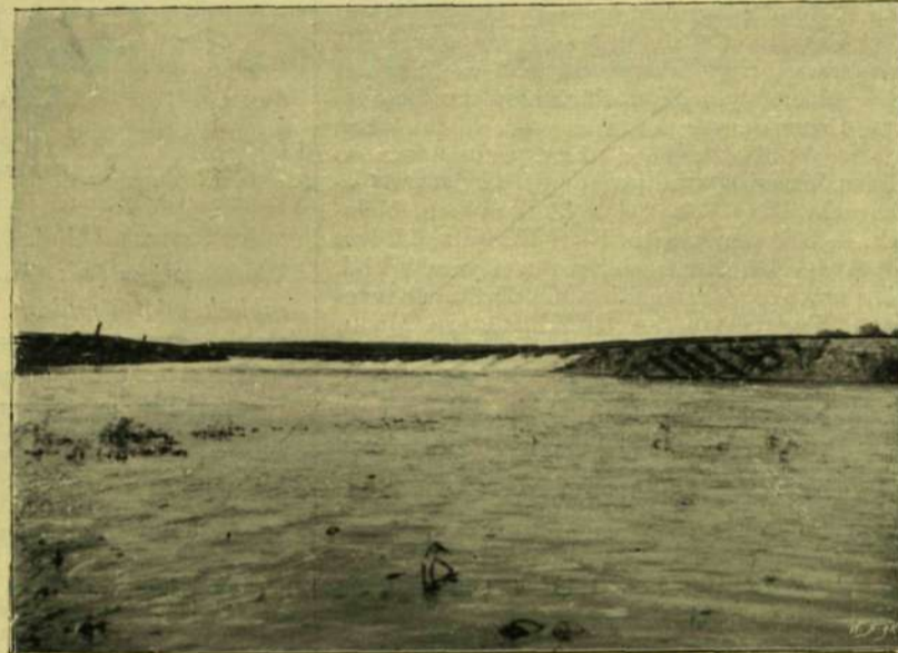
ÁRVIZ ÁLTAL ÁTSZAKÍTOTT VASUTI TÖLTÉS DUNA-ÚJFALU ELŐTT.
