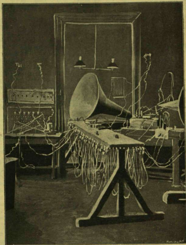
A TELEFON-HIRMONDÓ MŰSZAKI OSZTÁLYÁNAK KÍSÉRLETEZÉSI TERME.
