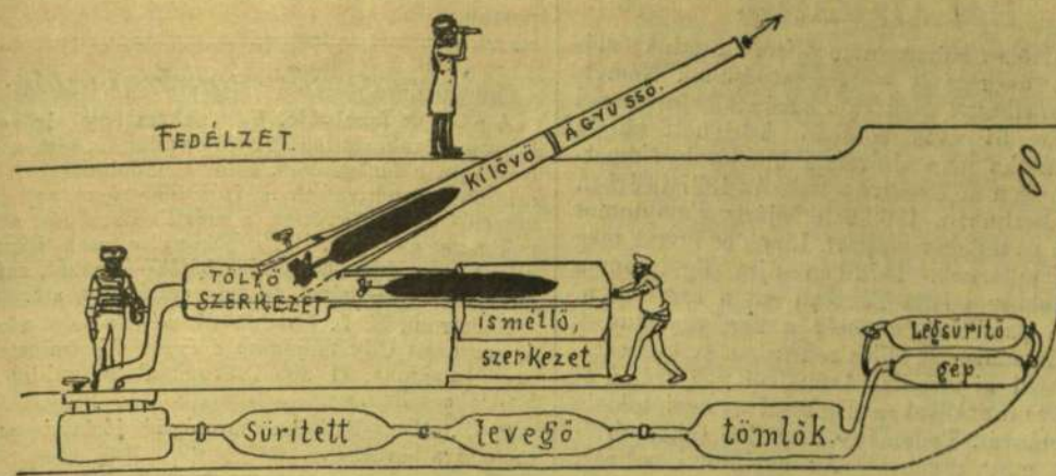
A «VESUVIUS» AMERIKAI DINAMIT-SZÓRÓ HAJÓ ÁTMETSZETE.
