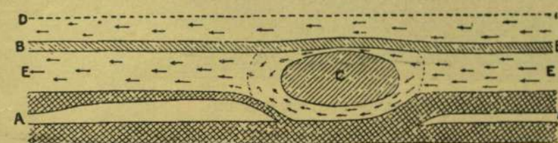
A «VÖRÖS FOLT» A JUPITEREN ÉS A LÉGKÖR ÁRAMLATAI.
