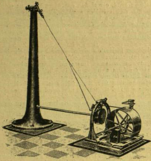
FÖLDRENGÉSJELEZŐ KÉSZÜLÉK. («A földrengések megfigyelése» cz. közleményhez.)
