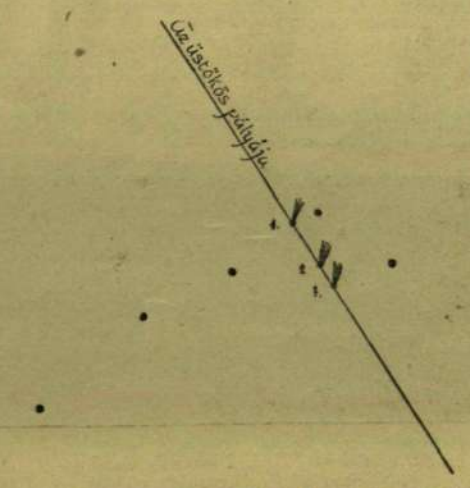
AZ ÚJ BORELLI-FÉLE ÜSTÖKÖS PÁLYÁJA. 1. Az üstökös július 28-án este 11 óra 30 perczkor, 2. július 29-én este 9 óra 15 perczkor, 3. július 30-án reggel 2 órakor.
