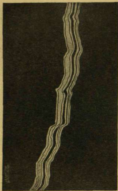
Közelről felvett lesújtó villám. Felvette ifj. Rümker G. Hamburgban 1898 aug. 16-án.
