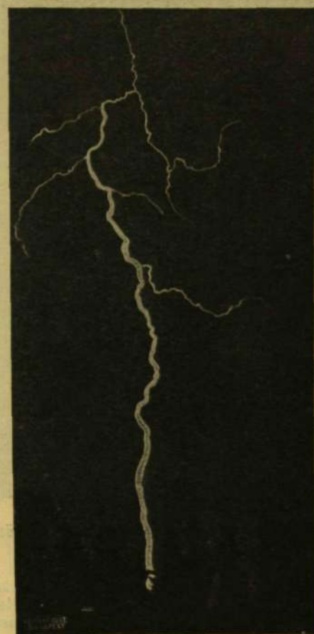
Lesújtó villám. Felvételtett Csillaghegyen 1901. július 23-án.
