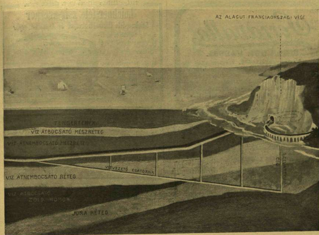
A CALAISAI CSATORNA ALATT TERVEZETT ALAGÚT ÁTMETSZETE. A tengerfenéki geológiai alakulata, az alagút irányával s vízlevezető csatornáival.
