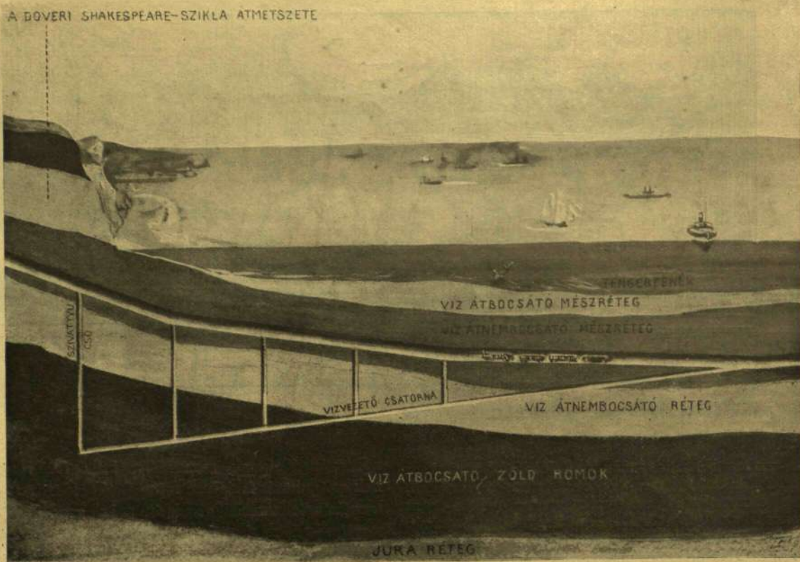
A CALAISAI CSATORNA ALATT TERVEZETT ALAGÚT ÁTMETSZETE. A tengerfenéki geológiai alakulata, az alagút irányával s vízlevezető csatornáival.
