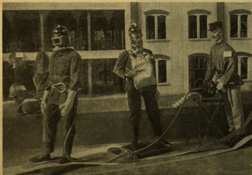
KÉSZÜLÉK, MELYNK SEGÍTSÉGÉVEL A TŰZOLTÓRAT ELLÁTJÁK LEVEGŐVEL.
