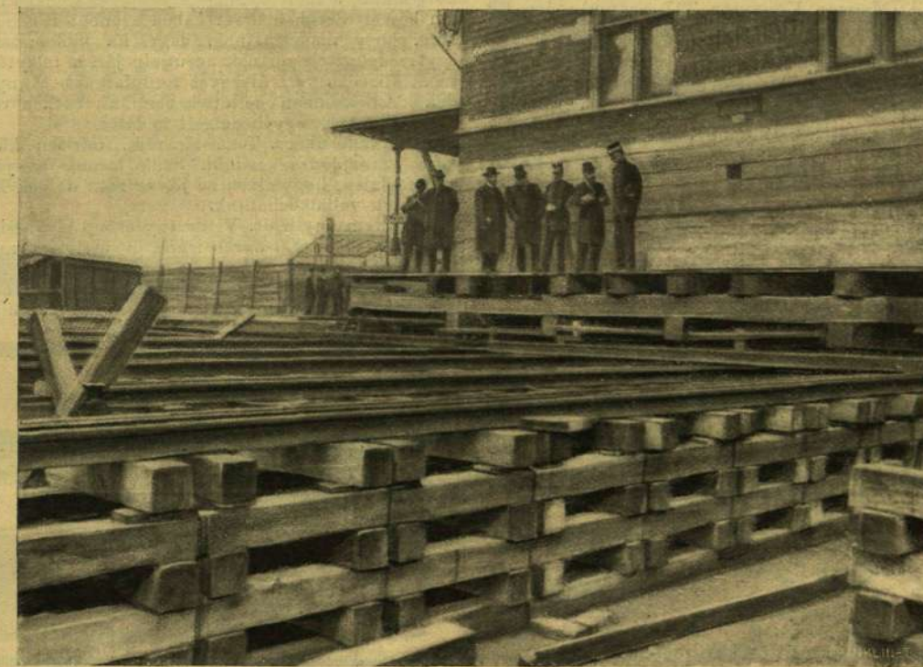
A PÁLYA, MELYEN AZ ÉPÜLETET ELTOLJÁK.
