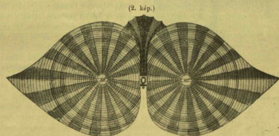
DÉGEN REPÜLŐ GÉPE FELÜLRŐL NÉZVE.
