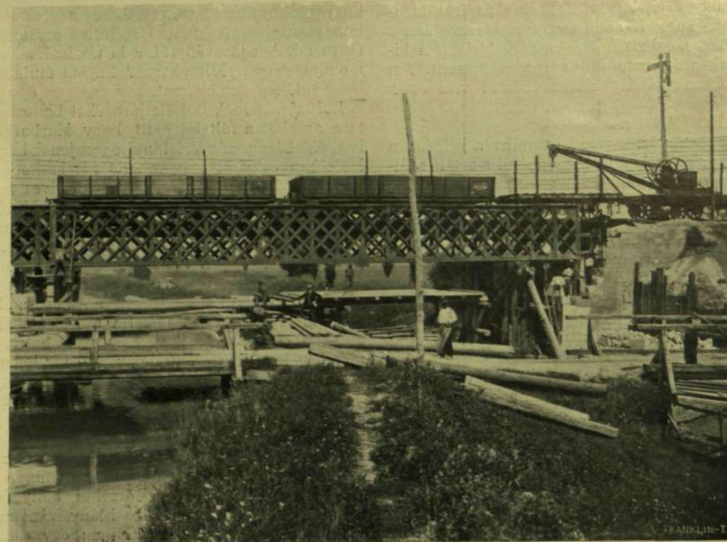
AZ ÚJ BALATONI VASÚT SZABADBATTYÁNI ÁTHIDALÁSA.
