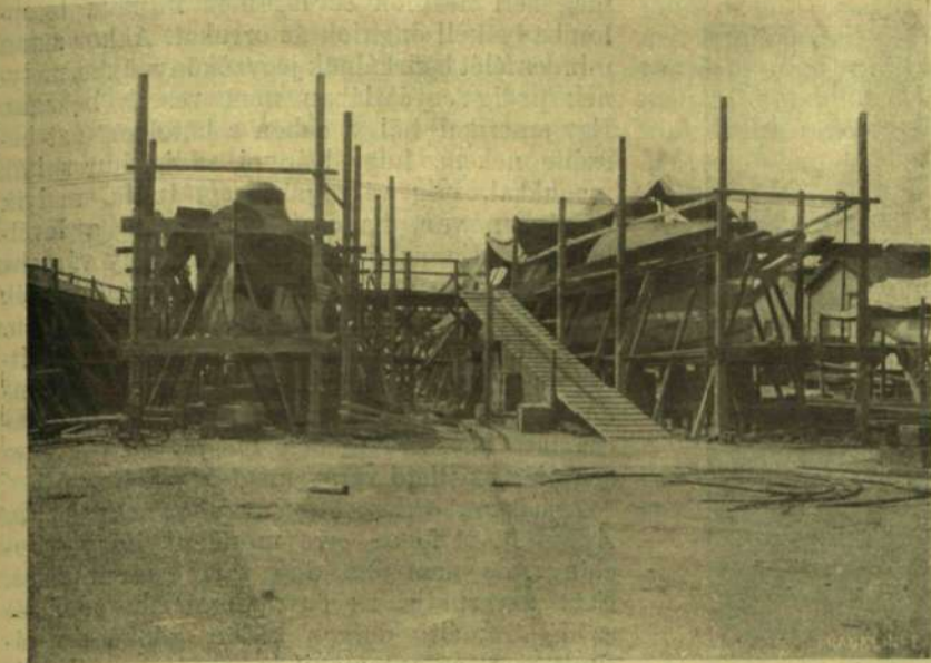
ÉPÜLŐ TORPEDÓ-NASZÁDOK.
