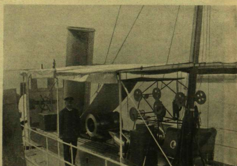
A „Gna” motollája, a melylyel 15,000 m. drót segítségével a sárkányokat és ballonokat a magasba bocsátják.
