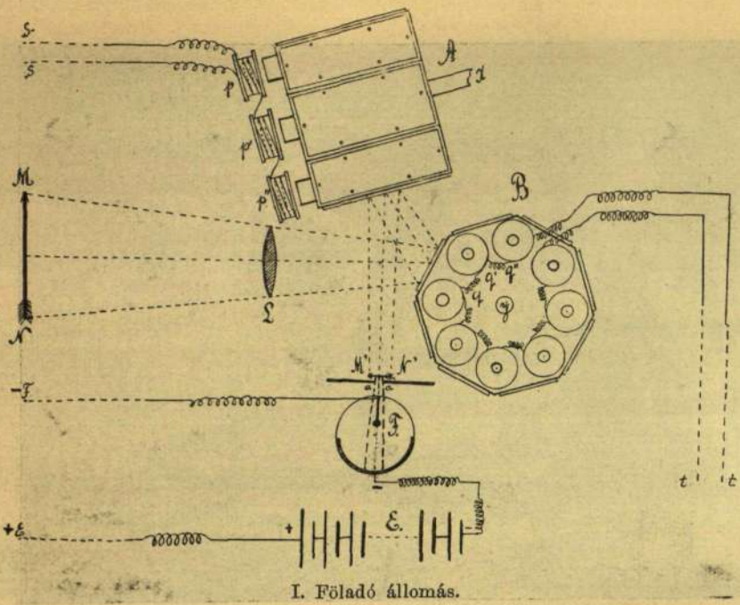
ROSIŃG TÁVOLBALÁTÓ KÉSZÜLÉKE.
