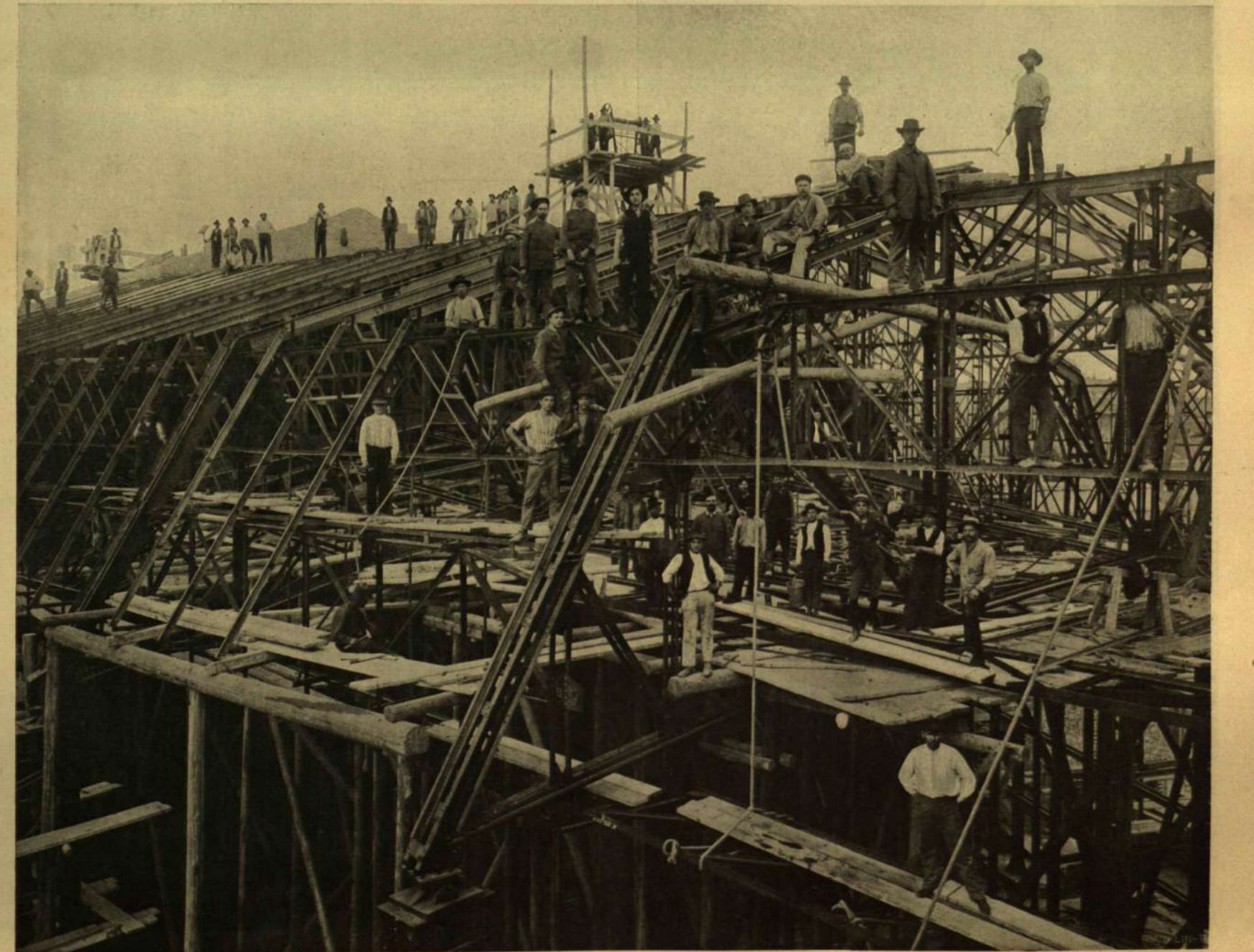
A FEDÉLSZERKEZET.
