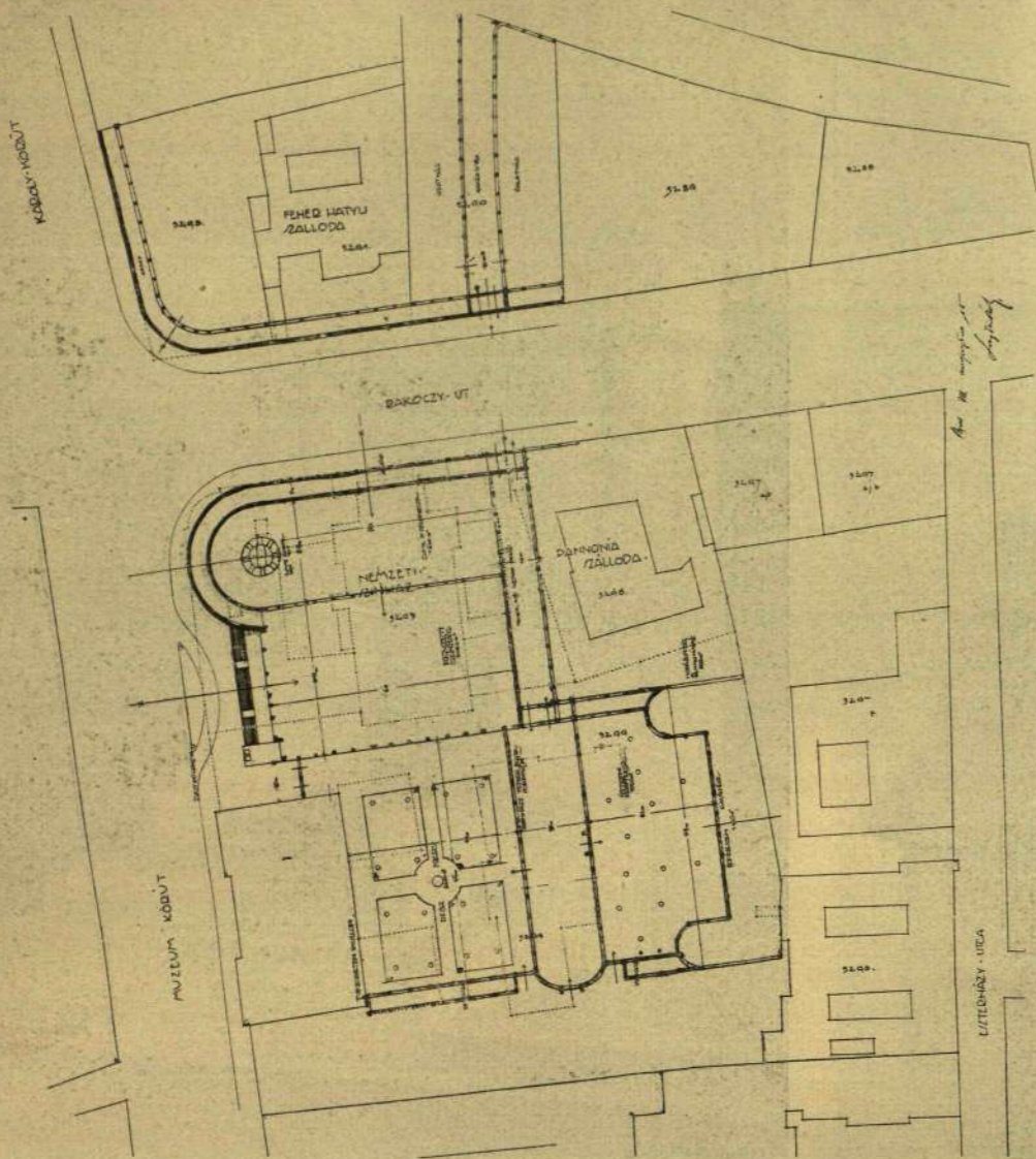
A Nemzeti Színház elhelyezési pályanyertes tervének alaprajza.
