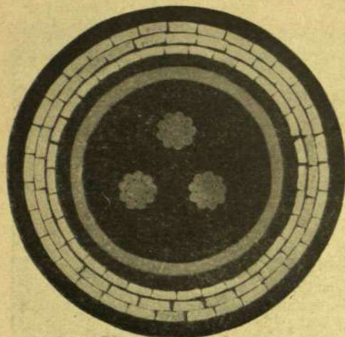
A kábel keresztmetszete természetes nagyságban.
