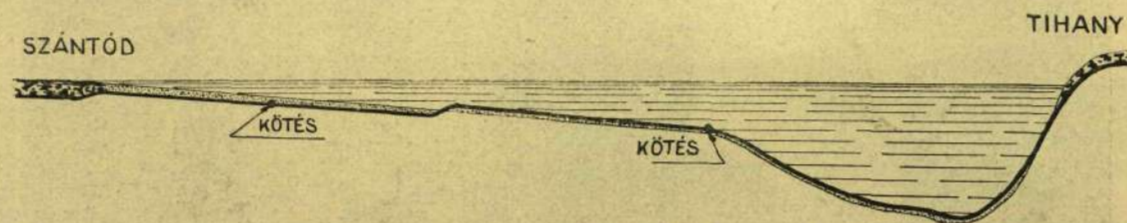
A BALATON KERESZTMETSZETE TIHANY ÉS SZÁNTÓD KÖZÖTT ELFEKTETETT KÁBELEKKEL.
