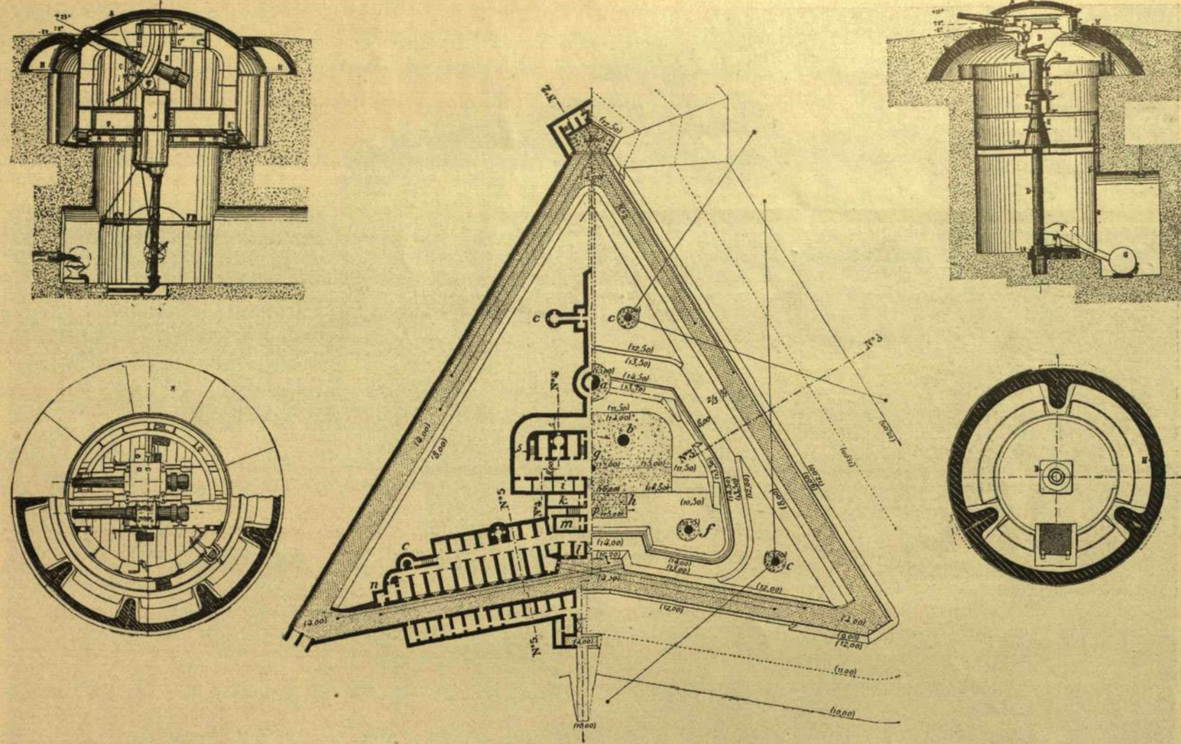
Forgatható és felemelhető páncéltorony 15 centiméteres ágyúkkal. — Az erődítmény alap és helyszínrajza. — Forgatható és felemelhető páncéltorony 5-7 centiméteres gyorstűzelő ágyúval.
