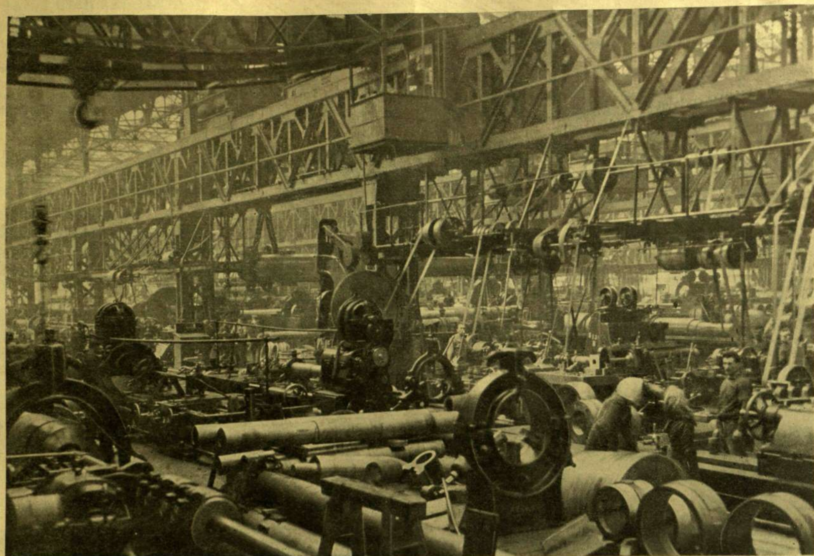
ÁGYESZTERGÁLYOZÁS.
