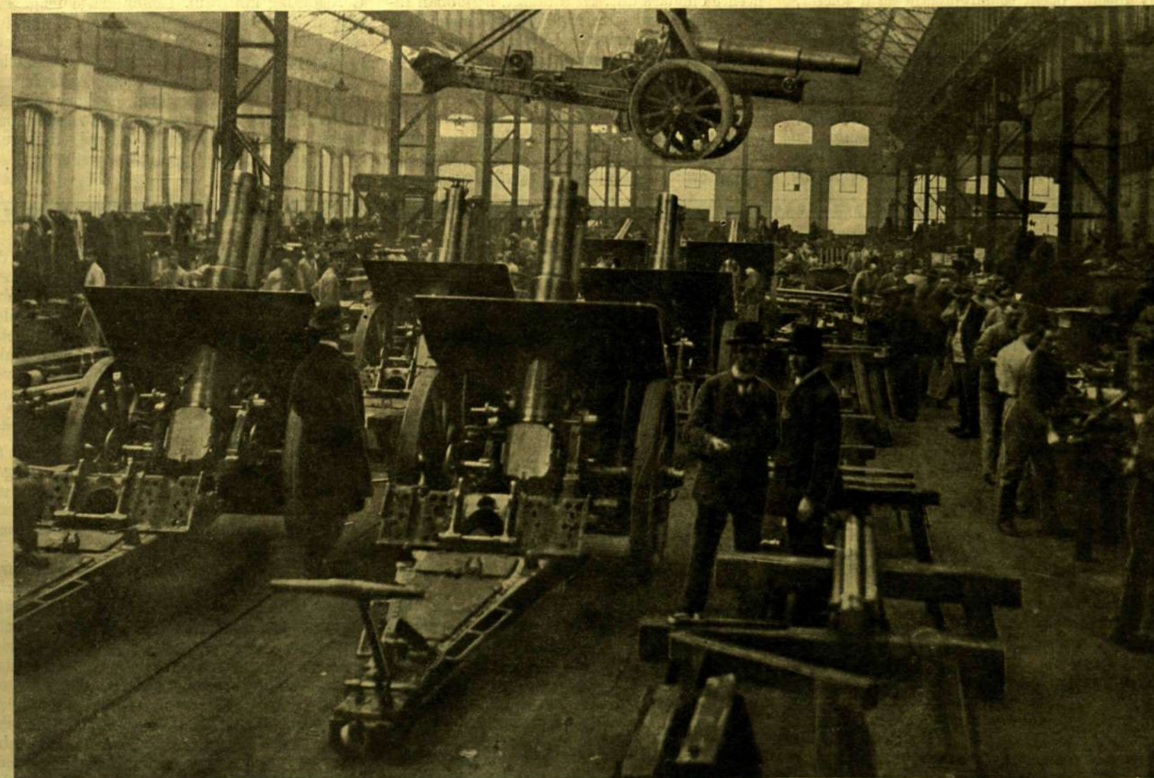
SZERELŐ-OSZAROK.
