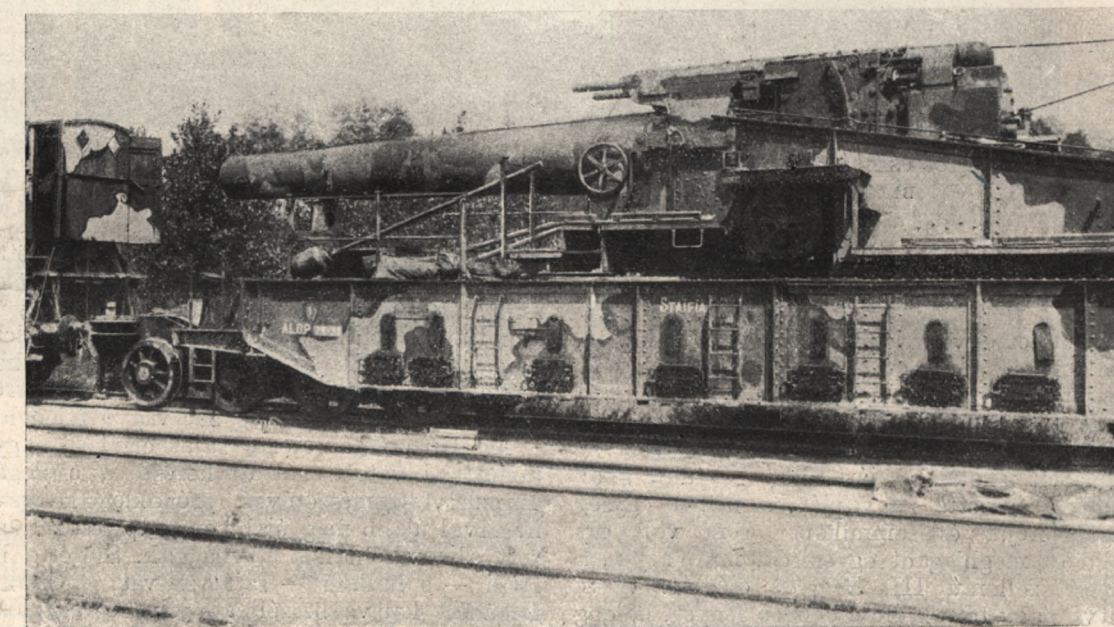
ZSÁKMÁNYOLT FRANCZIA VASUTI LÖVEG.
