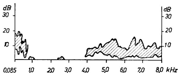
21. ábra A helyesen képzett sz hangok amplitudóinak alsó és felső burkológörbéje
