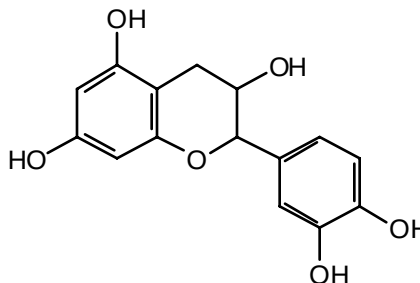
katechin
