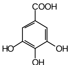
gallusz-sav: 3,4,5-trihidroxibenzoéssav
