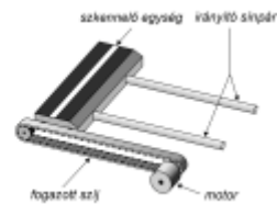
2. ábra Síkágyas szkennер vázlatos felépítése
