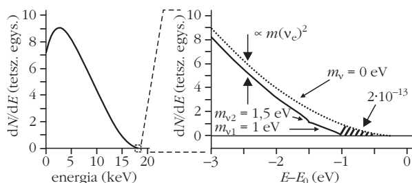
4. ábra. A \beta -spektrum deformációja a neutrínó nem-zérus tömege következtében (az eloszlást a bal oldali ábra maximális elektron-energiájának közvetlen környezetében kinagyítva mutatja a jobb oldali ábra).
