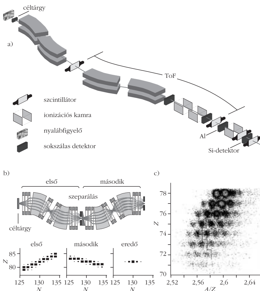
6. ábra. a) Fragmensszeparátor (FRS) a GSI-ben; a szeparált ionok implantálása Si-detektorokba. Az azonosítás kívül meghatározhatók a felezési idők is.
