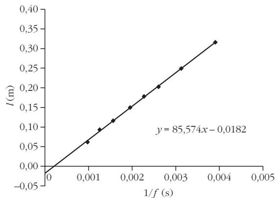
11. ábra. A d = 5,9 cm belső átmérőjű cső rezonanciagörbéje
