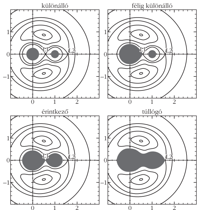
1. ábra. Gravitációs ekvipotenciális felületek kettőscsillagokban. Távolságegység a két csillag centrumának távolsága. L1, L2 az első és a második Lagrange-pont helyzete (az öt Lagrange-pont a pontosított testekből álló háromtest-probléma öt egzakt megoldásához kapcsolódik, az e pontok egyikébe helyezett harmadik próbatest és a két másik test mozgása önhasonló lesz). Az ábrákon rendre a különálló, félig különálló, érintkező és túllógó (közös burok) típusokat látjuk.
