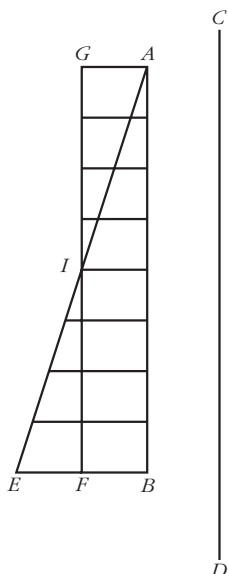
3. ábra. Galilei sebesség-idő függvénye lerajzolva és a Discorsi 170. oldalán
