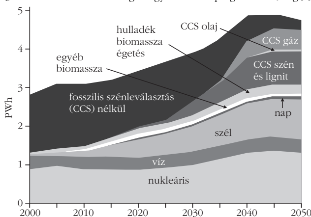
3. ábra. Az EU villamosenergia-fogyasztásának prognóza 2050-ig [8]
