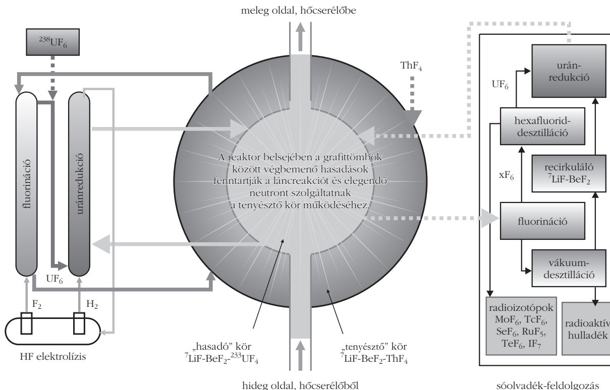
5. ábra. A kétkörös sóolvadékos tenyésztő működési vázlata [16].
