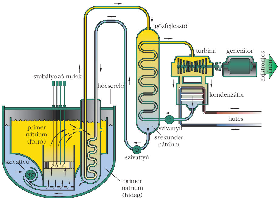
11. ábra. A nátriumhűtésű gyorsreaktor vázlata. Forrás: http://upload.wikimedia.org/wikipedia/commons/d/d8/Sodium-Cooled_Fast_Reactor_Schemata.svg
