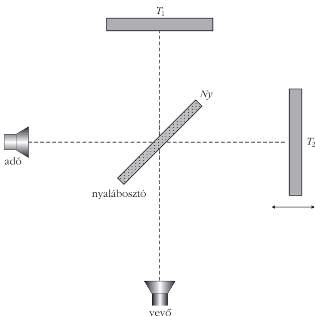
10. ábra. A Michelson-féle interferométer elvi vázlata.
