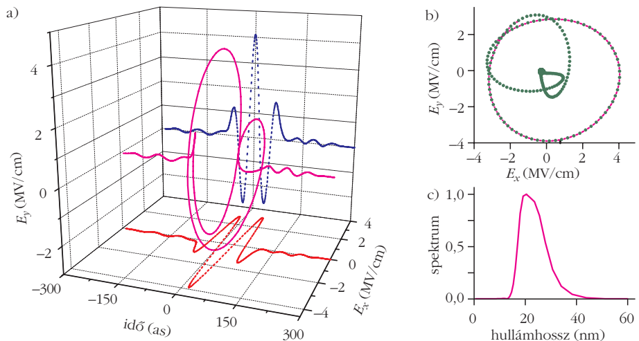
5. ábra. a) Cirkulárisan polarizált attoszekundumos impulzus időbeli lefutása (folytonos görbe), valamint x és y irányú komponense (pontosított vonal). b) Az elektromos térerősség időbeli változása az x - y síkon. c) A keletkező attoszekundumos impulzus intenzitás spektruma.
