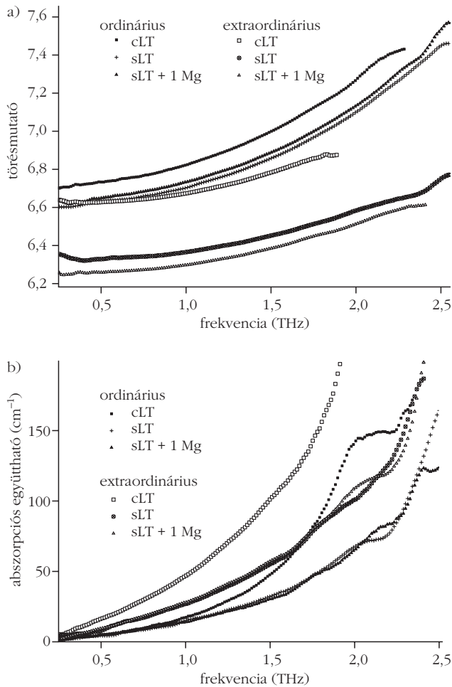
5. ábra. Adalékoltalan kongruens (cLT) és sztöchiometrikus (sLT), illetve 1 mol% Mg adalékolt sztöchiometrikus LT (sLT + 1 Mg) ordinárius és extraordinárius irányú frekvenciafüggő dielektromos jellemzői (fölső törésmutató, alul az abszorpciós együttható).
