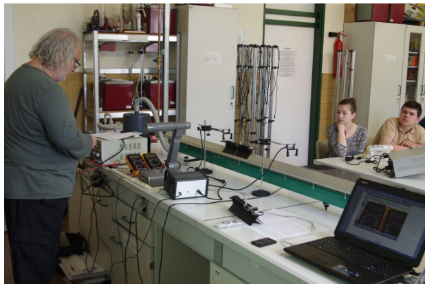
1. ábra. Az ütközések vizsgálatához használt sín-pálya, fotocapuk, időmérő.
