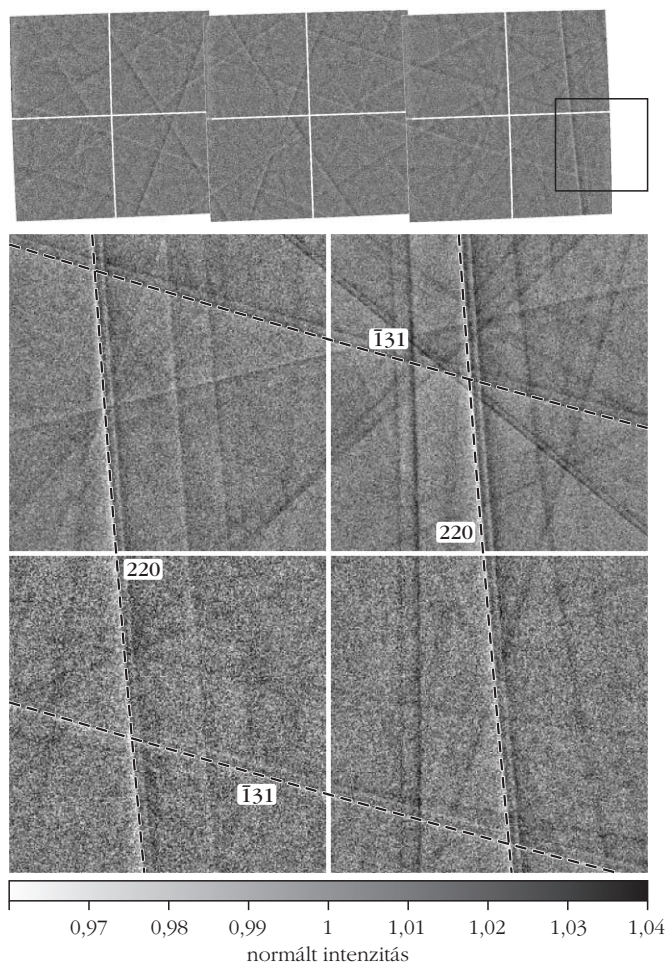
4. ábra. Egy GaAs egykristálymintán végzett mérés eredményei. Balra: a Kossel-vonalmintázat indexeléséhez felvett nagyobb térszögű összeillesztett mozaikkép és a fekete négyzettel jelölt részen nagyobb felbontással felvett kép néhány jellegzetes Kossel-vonal kiemelésével. A képen párhuzamosan futó azonos indexű vonalak (valójában koaxiális kúpok) a mintában előforduló kétféle forrásatom (Ga, As) 3-3 – K\alpha_{1,2} és K\beta – emissziós vonala, azaz a hatféle energia következménye. Jobbra: néhány kiválasztott példa a képből kinyert profilok és az elméleti görbék illeszkedésére a Kossel-vonal adatainak feltüntetésével.
