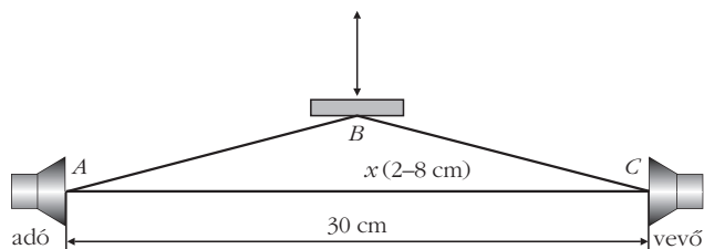
8. ábra. A Lloyd-féle tükörkísérlet.
