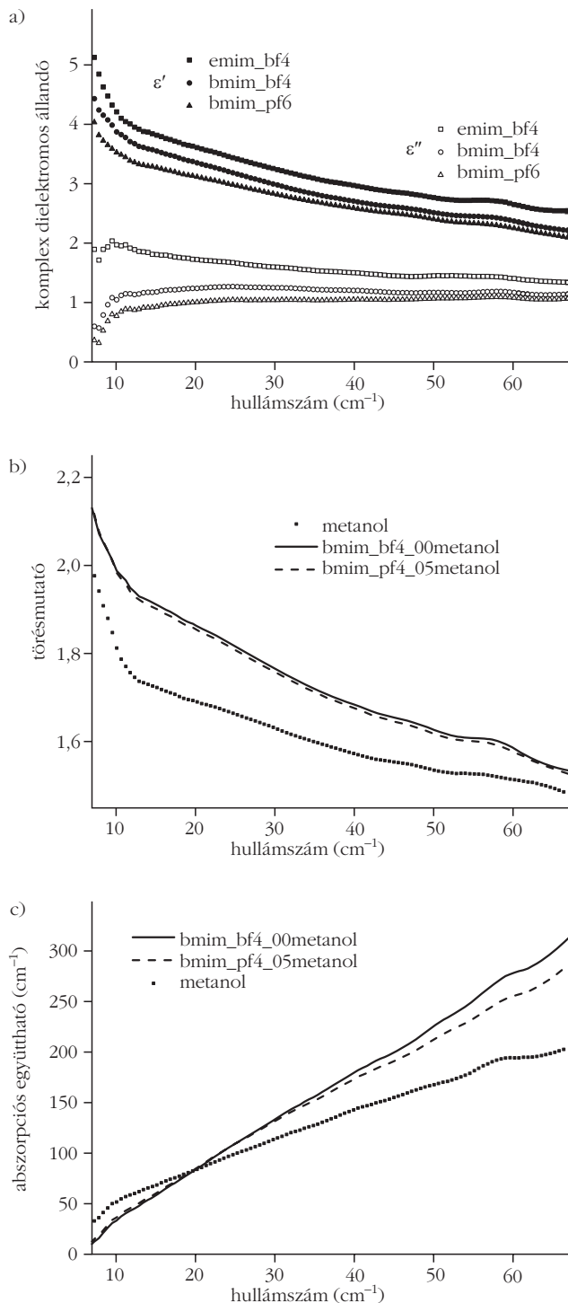
6. ábra. Ionfolyadékok dielektromos jellemzői (a: komplex dielektromos állandó, b: törésmutató, c: abszorpciós állandó). emim_bf4: etil-metil-imidazolium-tetrafluoroborát, bmim_bf4: butil-metil-imidazolium-tetrafluoroborát, bmim_pf6: butil-metil-imidazolium-hexafluorofoszfát.
