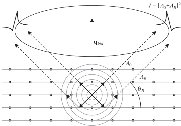
1. ábra. A Kossel-vonalak kialakulásának szemléltetése. A mintán belüli keltett gömbhullámforrások A_0 direkt sugárzása interferál ugyanezen sugárzás rácscsíkokra merőleges tengelyű kúpok mentén teljesül, amelyek egy síkdetektoron kúpszeletekként jelennek meg a síksereg mindkét oldalán. Ezek rendszere a kristály szimmetriájára és rácsparamétereire jellemző, intenzitásprofiljuk pedig a komplex szerkezeti tényezővel áll összefüggésben. A reflexió fázisára vonatkozó információt a kúpok mentén az interferencia következtében kialakuló intenzitásmoduláció, azaz a Kossel-vonalak szerkezete hordozza.
