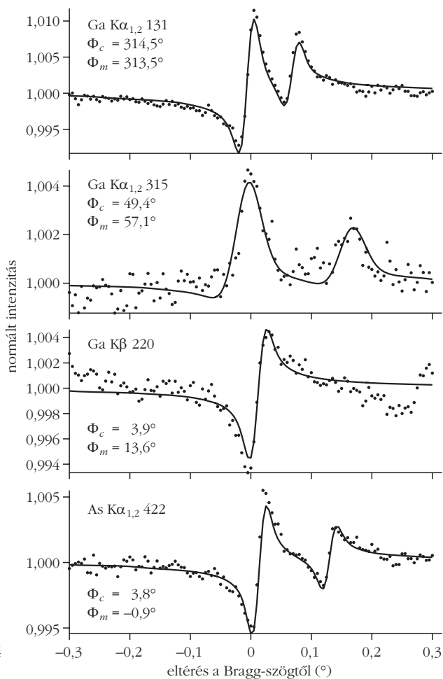
4. ábra. Egy GaAs egykristálymintán végzett mérés eredményei. Balra: a Kossel-vonalmintázat indexeléséhez felvett nagyobb térszögű összeillesztett mozaikkép és a fekete négyzettel jelölt részen nagyobb felbontással felvett kép néhány jellegzetes Kossel-vonal kiemelésével. A képen párhuzamosan futó azonos indexű vonalak (valójában koaxiális kúpok) a mintában előforduló kétféle forrásatom (Ga, As) 3-3 – K\alpha_{1,2} és K\beta – emissziós vonala, azaz a hatféle energia következménye. Jobbra: néhány kiválasztott példa a képből kinyert profilok és az elméleti görbék illeszkedésére a Kossel-vonal adatainak feltüntetésével.
