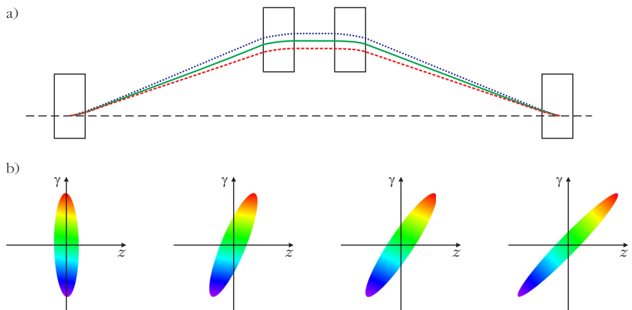
6. ábra. Fölül: a chicane és a rajta áthaladó különböző energiájú elektronok pályájának sématis rajza. Alul: a chicane-on való áthaladás különböző szakaszainál a fázistéren ábrázolt elektroncsomag.
