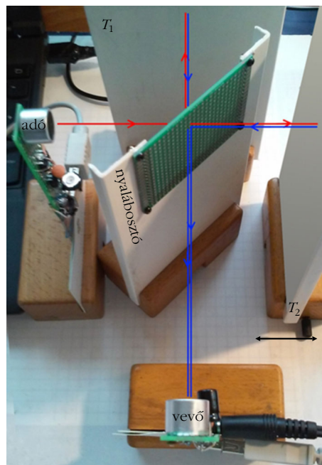
11. ábra. A Michelson-kísérlet fényképe.
