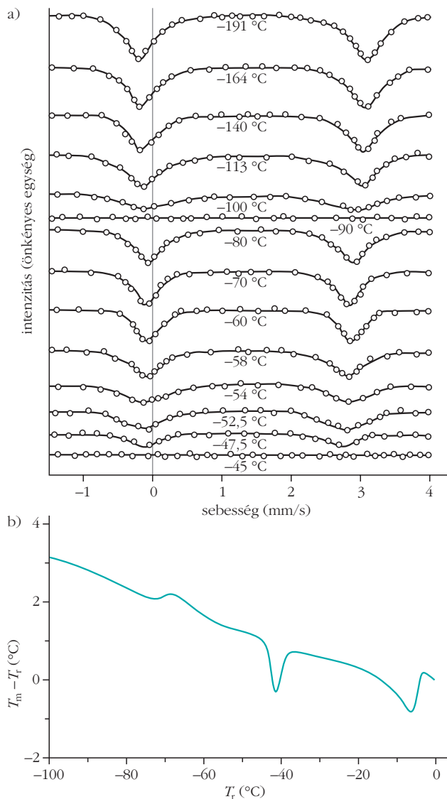
2. ábra. \text{Fe}(\text{ClO}_4)_3 lefagyasztott vizes oldata a) Mössbauer-spektrumainak és b) differenciális termoanalízisének hőmérsékletfüggése. T_m a minta, T_r pedig az inert referenciaanyag hőmérséklete.
