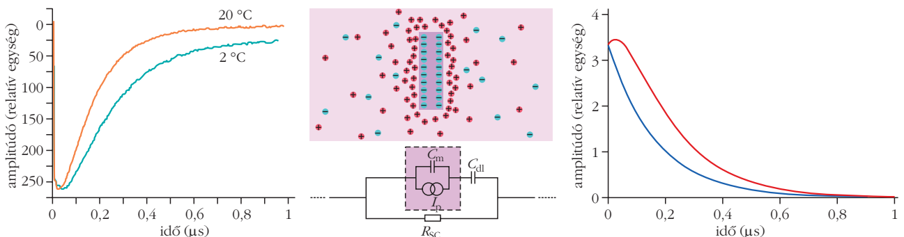
5. ábra. A membránon belüli gyors töltéssztérváltsást követő elektromos relaxáció két hőmérsékleten. A membrán-elektrolit rendszer sémája és egyszerűsített helyettesítő áramköre. I_p : áramgenerátor, C_m : membránkapacitás, C_{dl} : az elektromos kettősréteg kapacitása. Az elektródapáron mérhető jel kinetikája állandó, és változó C_{dl} mellett (kék, illetve piros görbe, rendre).
