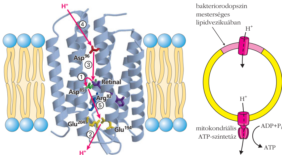
1. ábra. A sejtmembránban elhelyezkedő bakteriorodopszin-molekula főbb szerkezeti elemei; a Mitchell-hipotézis alátámasztása mesterséges lipidvezikulába ágyazott bakteriorodopszin és ATP-szintetáz segítségével [4].
