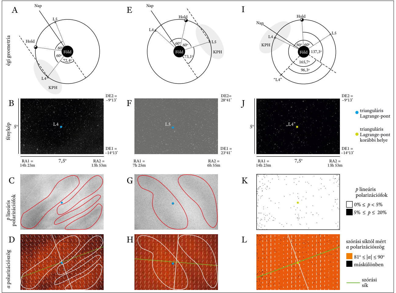
2. ábra. A Föld–Hold-rendszer L4 és L5 Lagrange-pontja körül Badacsonytördemecen képkalkotó asztropolarimetriával észlelt Kordylewski-féle porholdak (KPH) égi geometriája, valamint p lineáris polarizációfokának és \alpha polarizációs szögének mintázatai a Hold keringési síkjában. (A–D) 22:00:34 GMT (greenwichi középido); 2022. július 3.; a porhold fázisa: 65%; fázisszög: 72,4°; epocha: 2000,0; képközép: RA (rektaszenczió) = 14 óra 11 perc 3,89 másodperc; DE (deklináció) = -11^{\circ} 39' 10,65'' . (E–H) 23:02:52 GMT; 2021. október 31.; a porhold fázisa: 65%; fázisszög: 73,1°; epocha: 2000,0; képközép: RA = 7 óra 9 perc 26,57 másodperc; DE = 26^{\circ} 9' 40,3'' . Az L4 és L5 pontok helyét kék pontok jelölik. Az \alpha -mintázatokon a fehér pálcikák a helyi polarizációirányt mutatják. A zöld szórási síkra merőleges irányt a fehér egyenes szemlélteti. A porholdak főbb foltjainak körvonalát piros, illetve fehér zárt görbék jelzik a p - és \alpha -mintázatokon. A p - és \alpha -mintázatokon az egymásra merőleges fehér és zöld egyeneseken túli vonalak műholdak nyomai. (I–L) 20:14:51 GMT; 2022. július 24.; fázisszög: 96,3°; epocha: 2000,0; képközép: RA = 14 óra 11 perc 3,89 másodperc; DE = -11^{\circ} 39' 10,65'' ), amikor az L4 pont nem volt ebben az égi ablakban, ezért „L4” az L4 pont 2022. július 3-i 22:00:34 GMT időpontbeli helyét jelöli [8]
