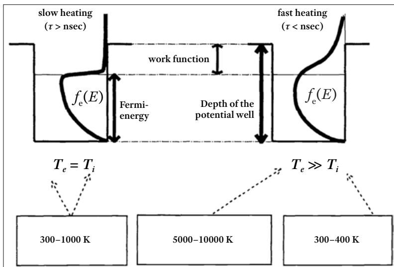
2. ábra. A termikus elektronemisszió típusai lassú fűtés és nem egyensúlyi, ultragyors felmelegítés hatására. Az elektronok f_e(E) Fermi-eloszlását a fém potenciálgödörében a vas-tag görbék jelképezik mindkét esetre, a függőleges tengelyen az energia. T_e és T_i az elektrongáz ( T_e ), illetve az ionrács ( T_i ) „pillanatnyi”, önmagával egyensúlyban lévő rendszerként értelmezett hőmérsékletének értékeit jelentik
