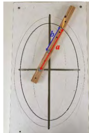
4. ábra. Ellipszográf
