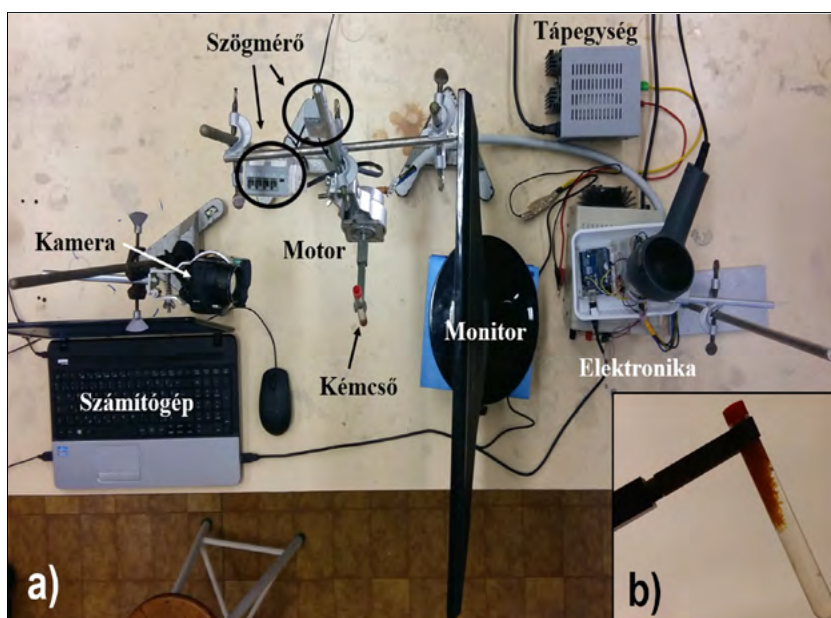
7. ábra. a) I. kísérleti eszközünk, b) fénykép az elemzett videóból
