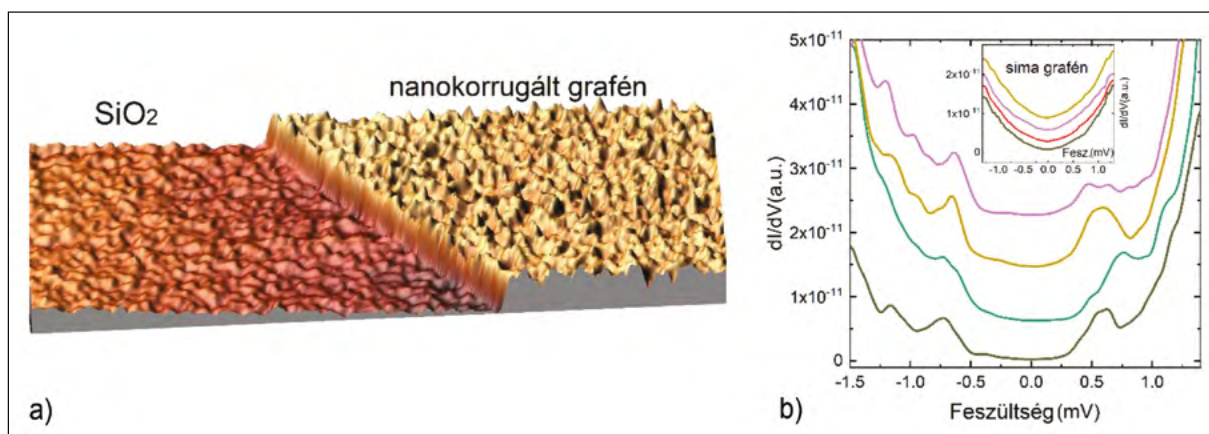
1. ábra. a) A ciklikus hőcsokkokkal meggyűrűt grafén AFM-képe minden korábbinál erősebb nanoskálájú gyűrődéseket (kb. 5 nm laterális méret, 1 nm magasság) mutat. b) Alagútspektroszkópiai mérések grafén gyűrődéseken jól azonosítható csúcsokkal (0,5 és 1 eV környékén), amelyek a töltéshordozók kvantumos bezártságát mutatják. Összehasonlításképp, a kvázisima grafénon mért alagútspektrumok nem mutatnak csúcsokat
