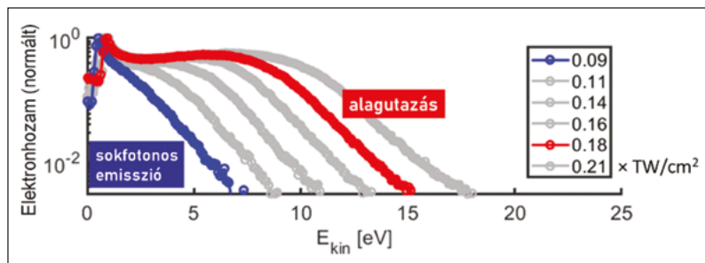
4. ábra. Tipikus fotoelektron-spektrumok alacsony lézerintenzitásoknál, ahol a sokfotonos emissziós mechanizmus dominál (kék görbe) és magasabb lézerintenzitásoknál, ahol az elektronok többsége alagutazással lép ki a felületről (vörös görbe)
