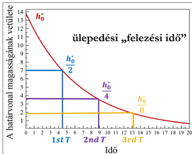
6. ábra. Az ülepedési felezési idő szemléltetése (sematikus ábra), a tengelyeken feltüntetett számok tetszőleges egységben vannak megadva
