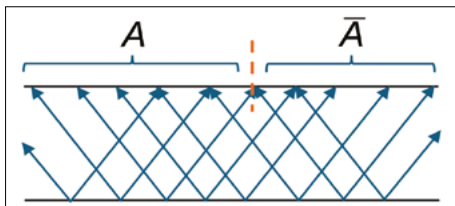
3. ábra. A korrelációk fejlődése a kvantumkvencs után, téridődiagramon szemléltetve, ahol az idő függőlegesen alulról felfelé telik. A nyilak a lokálisan keltett, egymással ellentétesen mozgó kvázirészecskékből álló párokat jelzik, az egyszerűség kedvéért mindegyiket ugyanazzal a sebességgel tüntettük fel. Az összefonódást azon párok növelik, amelyeknek egyik tagja az A , a másik pedig az \bar{A} tartományba érkezik; ezek száma az idő lineáris függvénye
