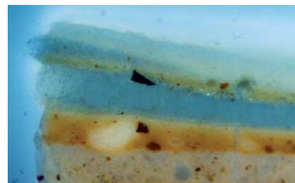
12. b. kép. A T5-ös minta keresztmetszet csiszolatának lumineszcens felvétele (450x). Legalább 4 (esetleg 5) eltérő lakkréteg különböztethető meg. A legkorábbi lakk, mely felett szennyeződé nyomok is láthatók, már csak nyomokban maradt meg.
