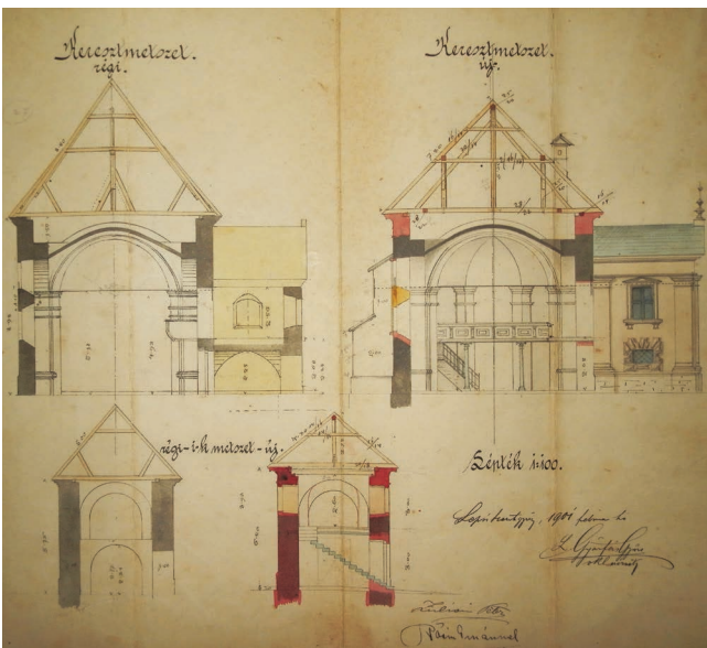
11. kép. A középajtai templom átalakítási tervei 1901-ből (a szerző felvétele (2017), forrás: Középajtai Református Egyház Levéltára, a terveket készítette: Gyárfás Győző, Sepsiszentgyörgy, 1901).
