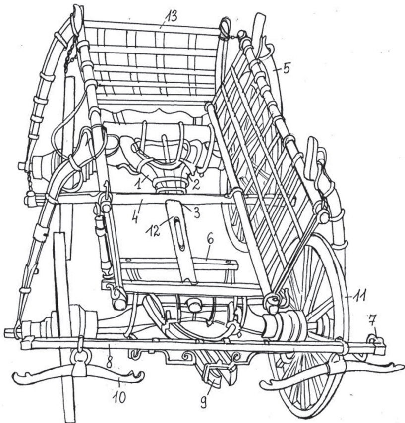
A szekér alváza: 1,2. nyújtószárny, 3. derékszeg, 4. hátulsó felhérc, 5. löcs, 6. fergettyű, 7. felhércvasalás, 8. első felhérc, 9. rúdszárny, 10. hámfá, 11. szekerkerek, 12. nyújtó, 13. hátulsó saroglya. (Rajz: Kész B.)
