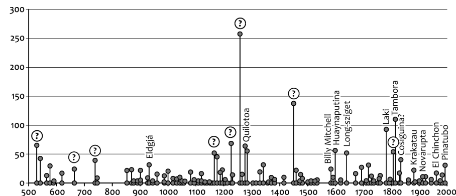
4. ábra • Az elmúlt 1500 év nagy vulkánkitörései, amelyek nyomot hagytak a grönlandi vagy antarktiszi jégtakaróban. A jégfuratmintákban mért savkoncentráció alapján becsülhető a sztratoszférába adott évben bekerült vulkáni kén-dioxid-gázokból keletkezett kénsav aeroszolmennyisége. Az anomális kénsavmennyiséghez köthető vulkáni kitörés vulkanológiai adatok hiányában sok esetben még nem ismert. A jégfuratminták ezért pontosabban dokumentálják a nagy vulkánkitörések számát (adatok Gao et al., 2008 alapján).
